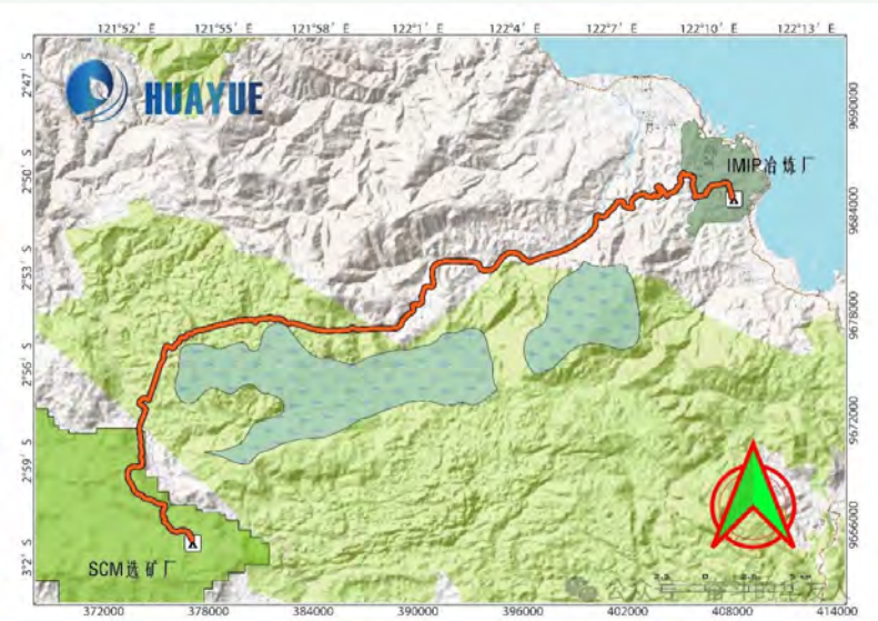
矿浆管线线路图
